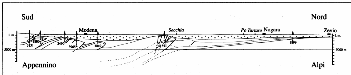
Fig. 11 - Struttura profonda della Pianura Padana in un profilo Nord-Sud. I depositi rappresentati dal retino puntinato sono quelli quaternari (da Pieri e Groppi, 1981).
